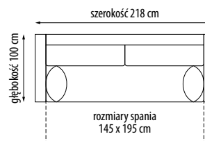
Schemat rozkładania funkcji spania typu DL
